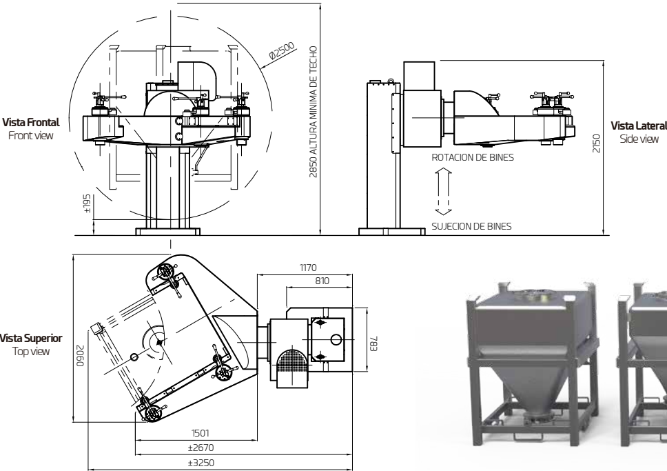
Brazo de acople con guías Quick coupling system
